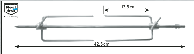
Spieß mit 2 Fleischklammern
