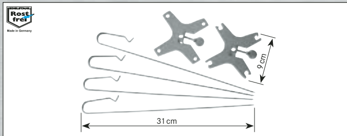
Fleischhalter 4 Spieße
