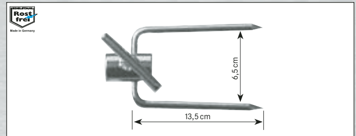
Fleischklammer
