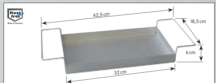
Fettauffangschale Edelstahl gebeizt
