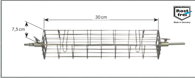
Fleischkorb Edelstahl
